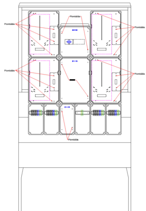
ELRENDEZÉSI RAJZ PLOMBÁLÁSI HELYEKKEL (kizárólag jó minőségű):
